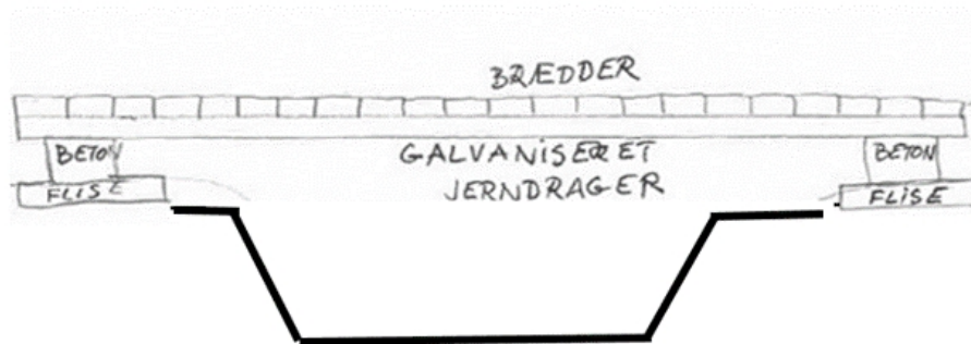
Figur 2: Principskitse for bro over Skovfenne Bæk.
